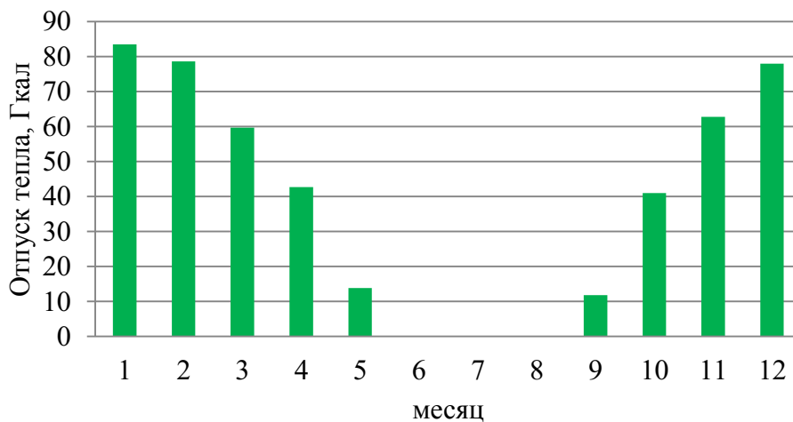
Рисунок 1.12 – Оптимальный температурный график отпуски тепловой энергии для котельной с. Новоколомино
