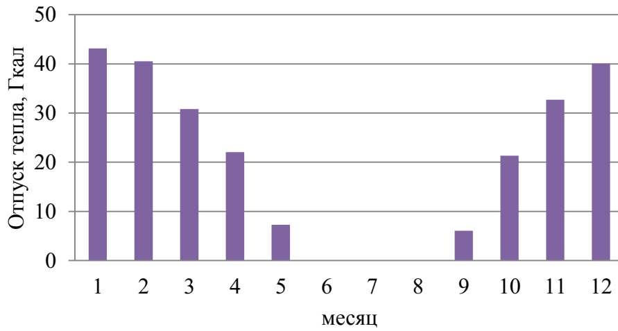
Рисунок 1.10 – Оптимальный температурный график отпуски тепловой энергии для котельной №1 с. Леботер
