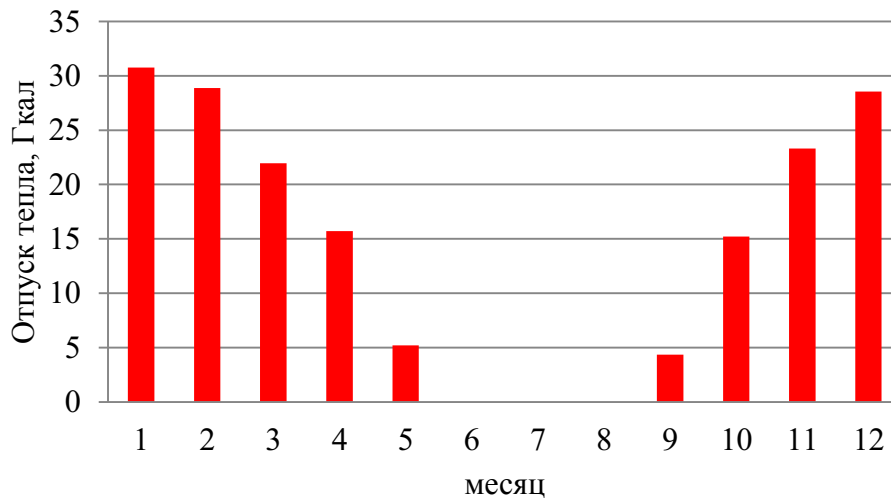
Рисунок 1.11 – Оптимальный температурный график отпуски тепловой энергии для котельной №2 с. Леботер
